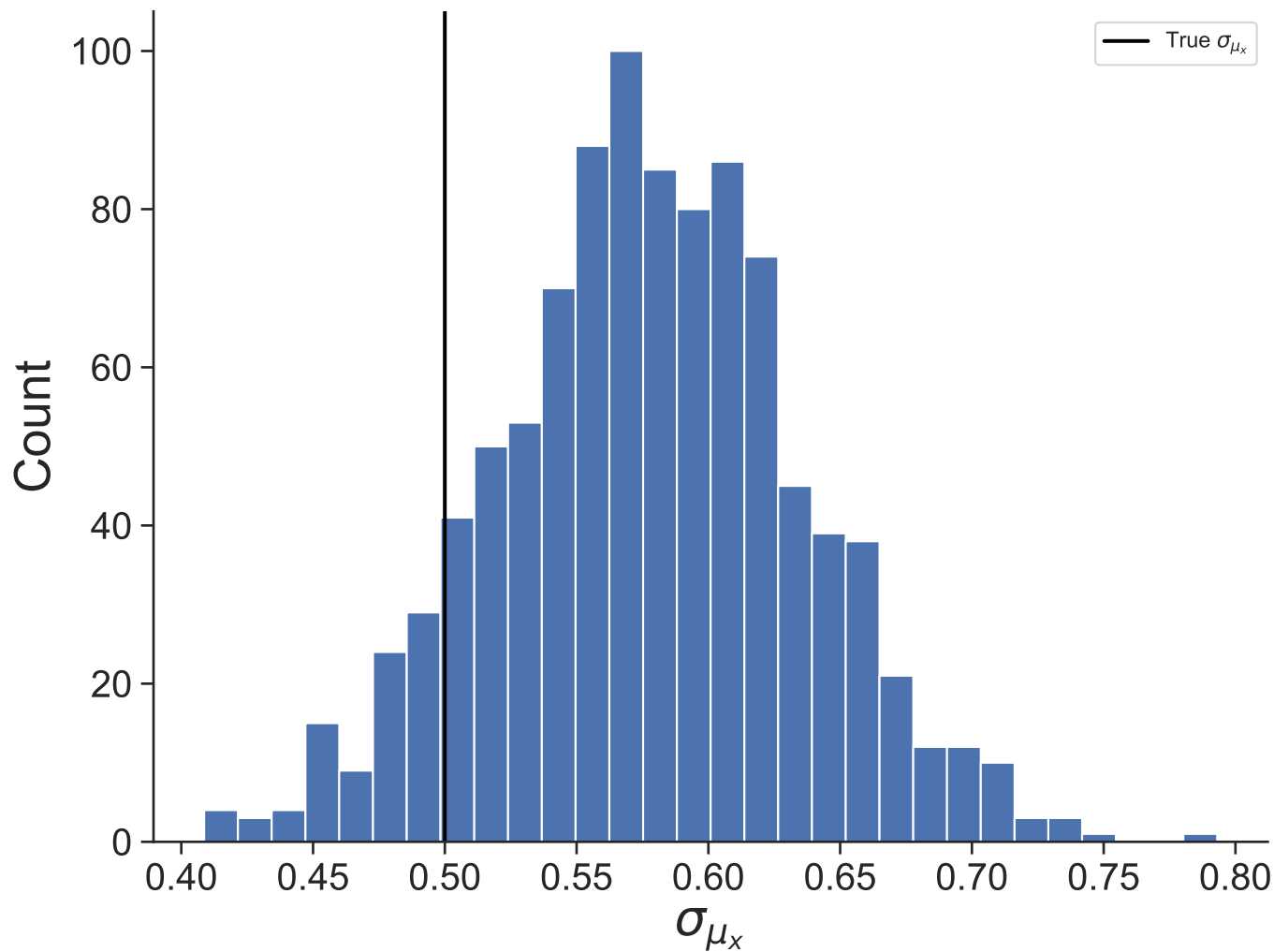
Dataset 12
