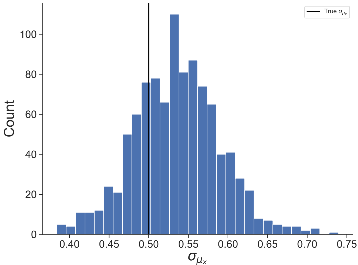
Dataset 31
