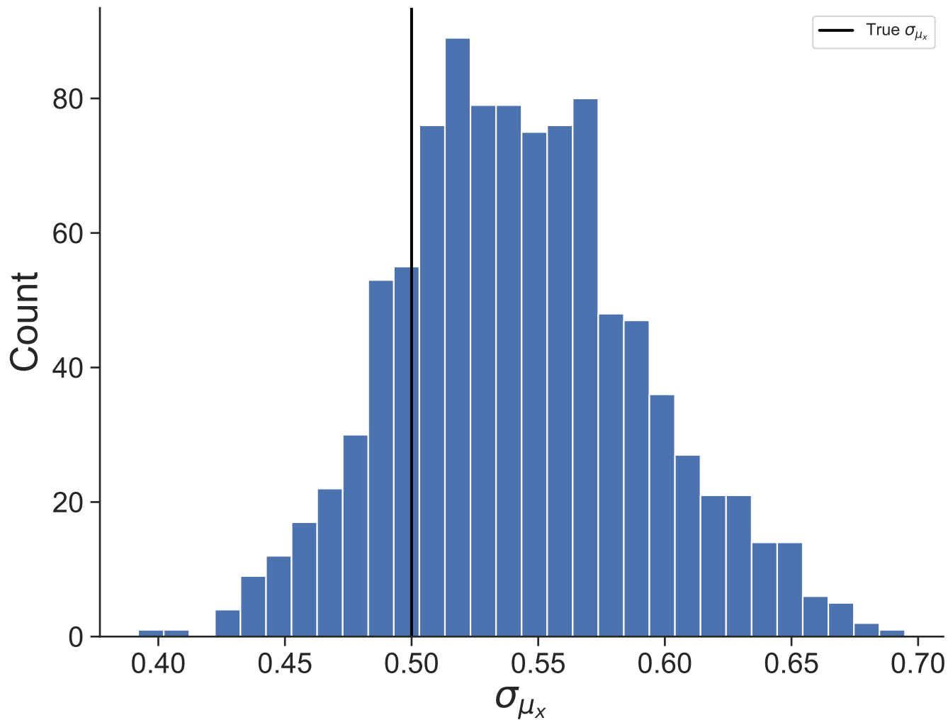
Dataset 42
