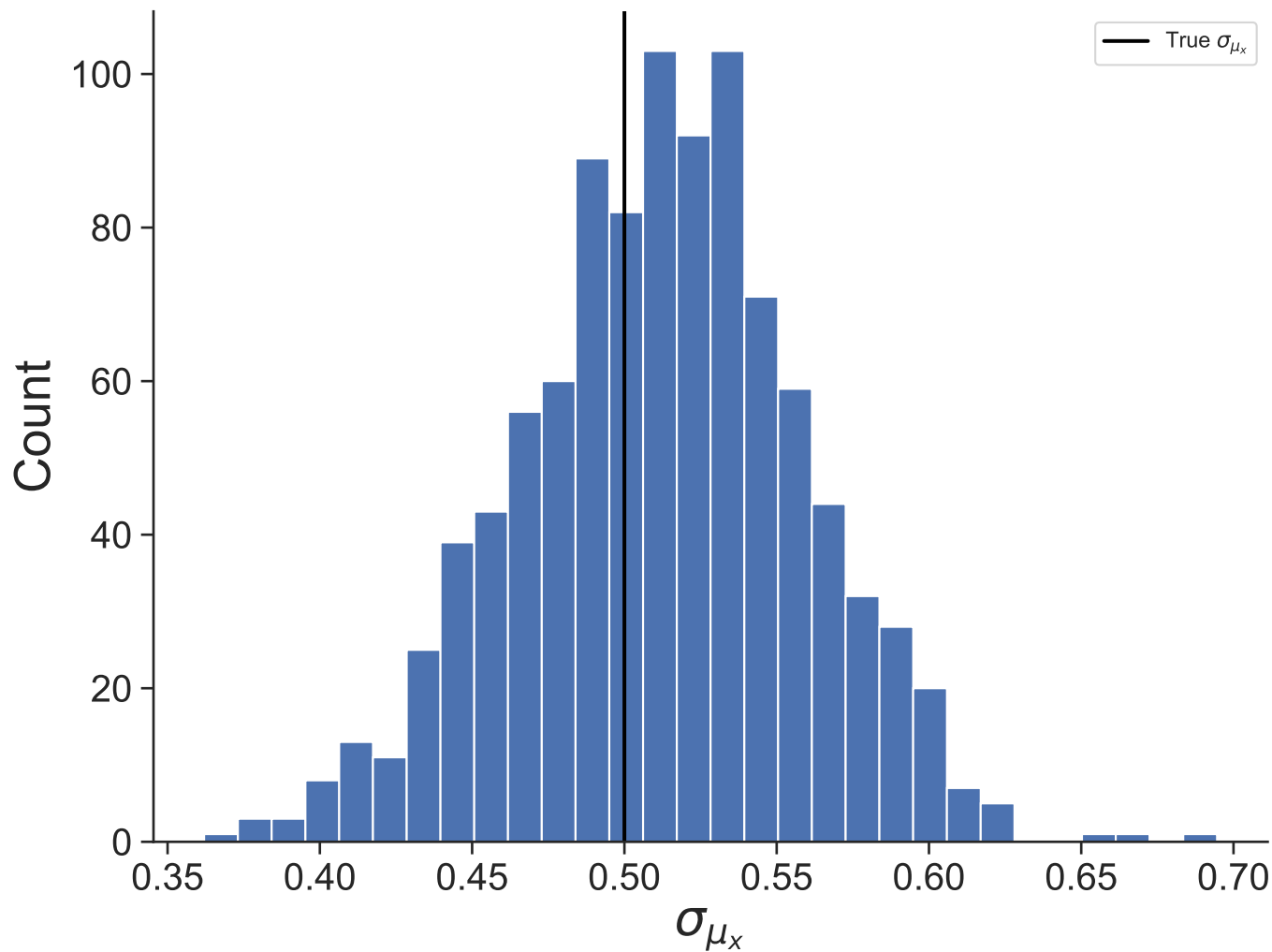
Dataset 4
