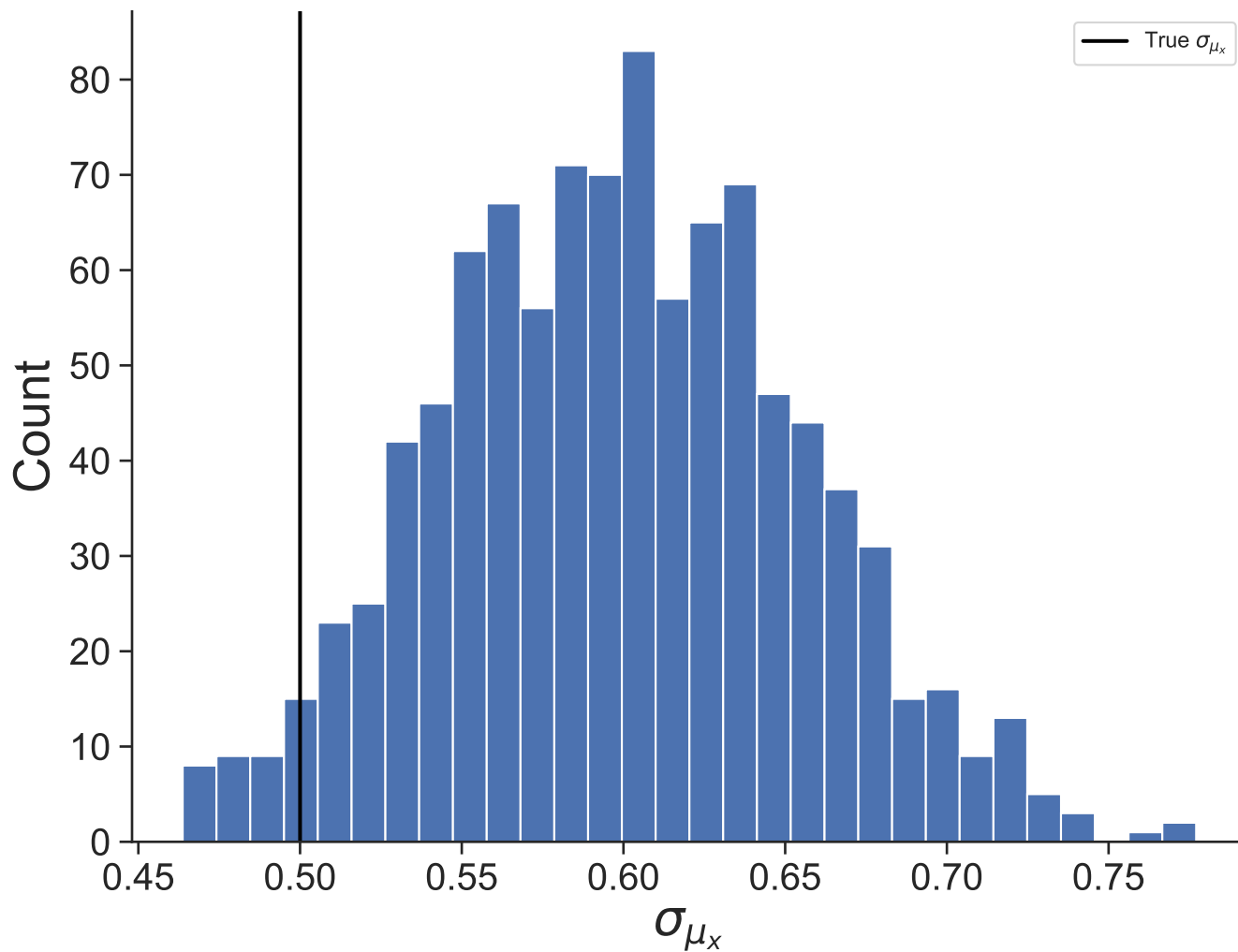
Dataset 1
