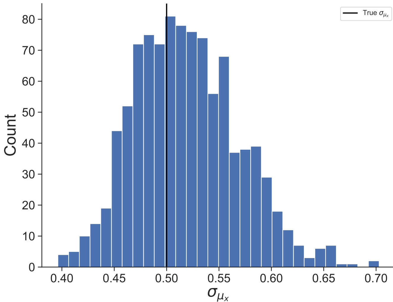
Dataset 11
