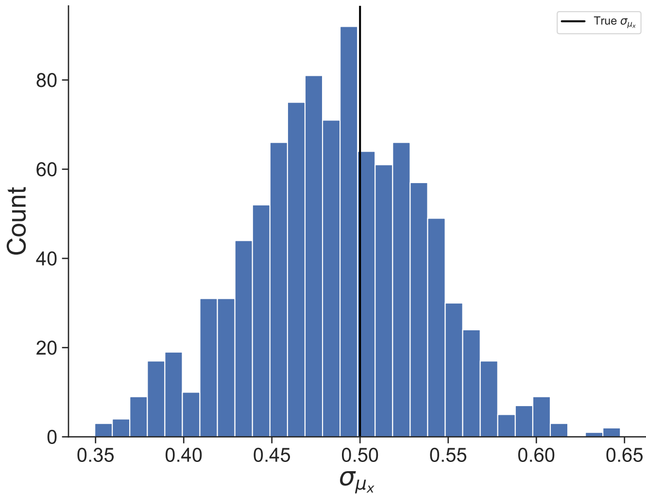
Dataset 40
