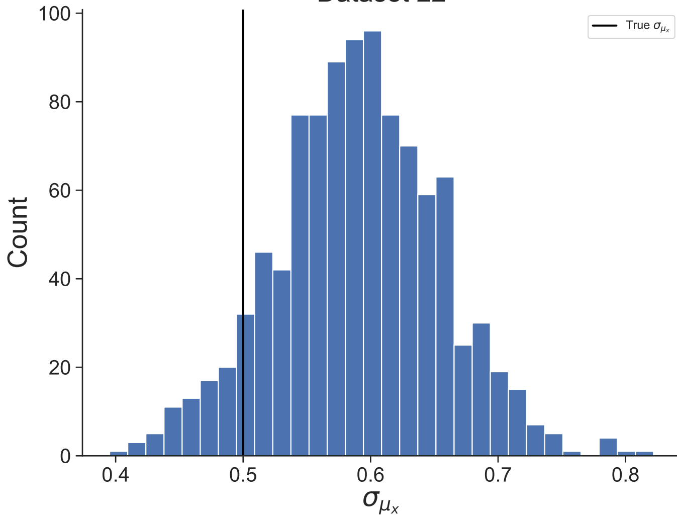
Dataset 22
