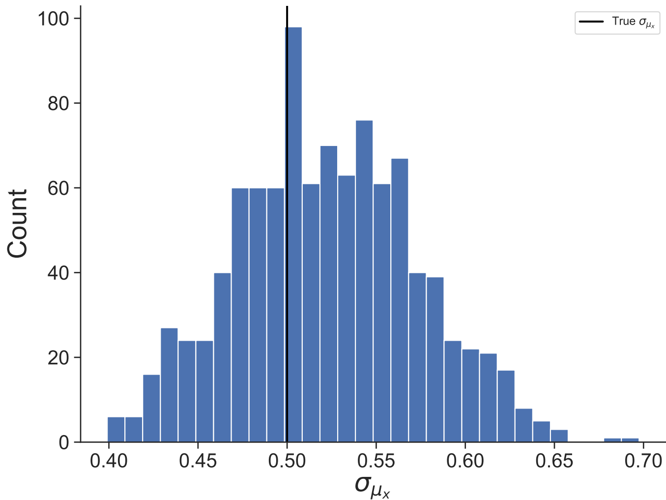
Dataset 5
