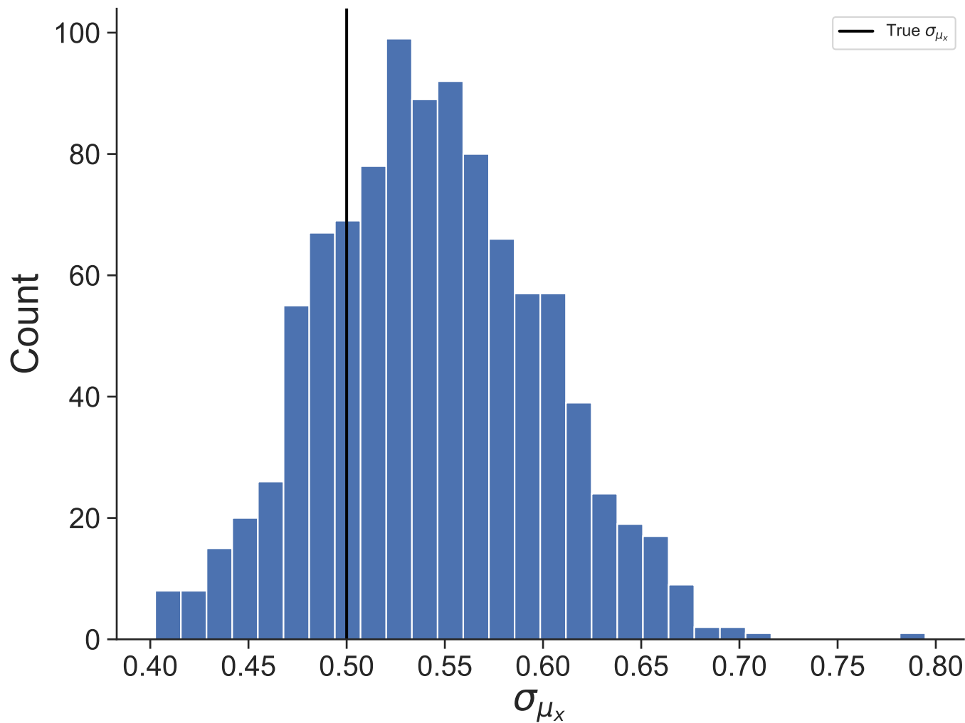
Dataset 32
