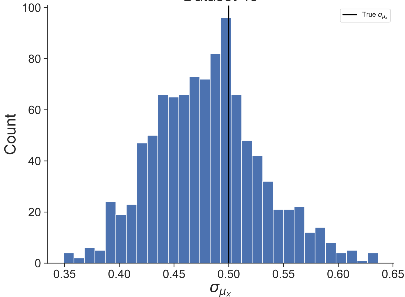
Dataset 43
