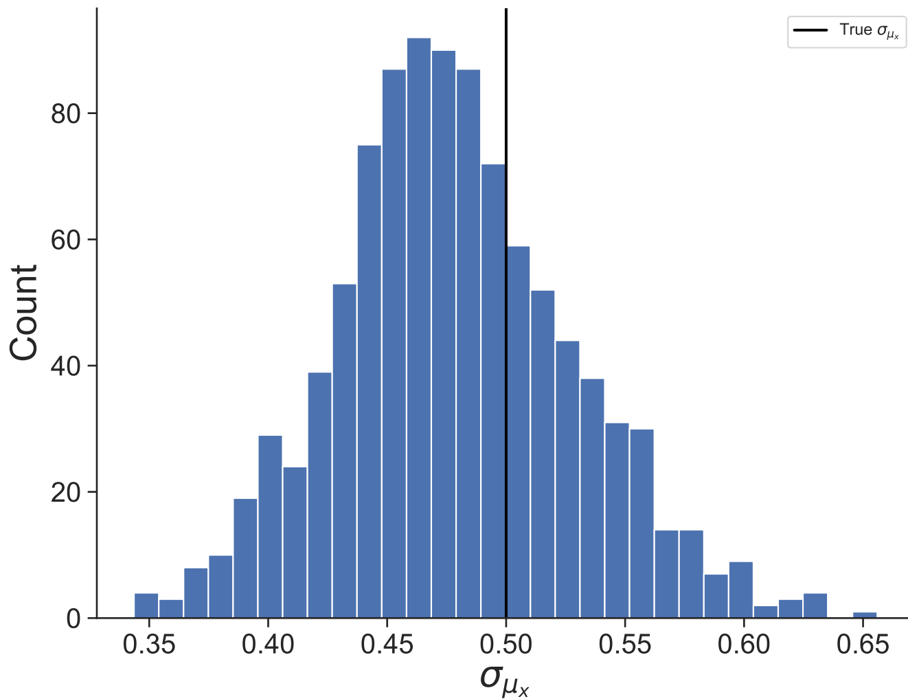
Dataset 45
