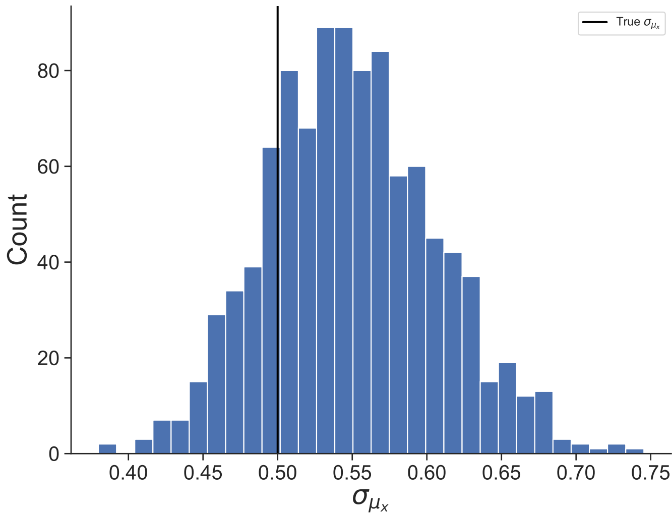
Dataset 27
