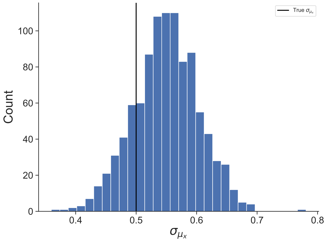
Dataset 16
